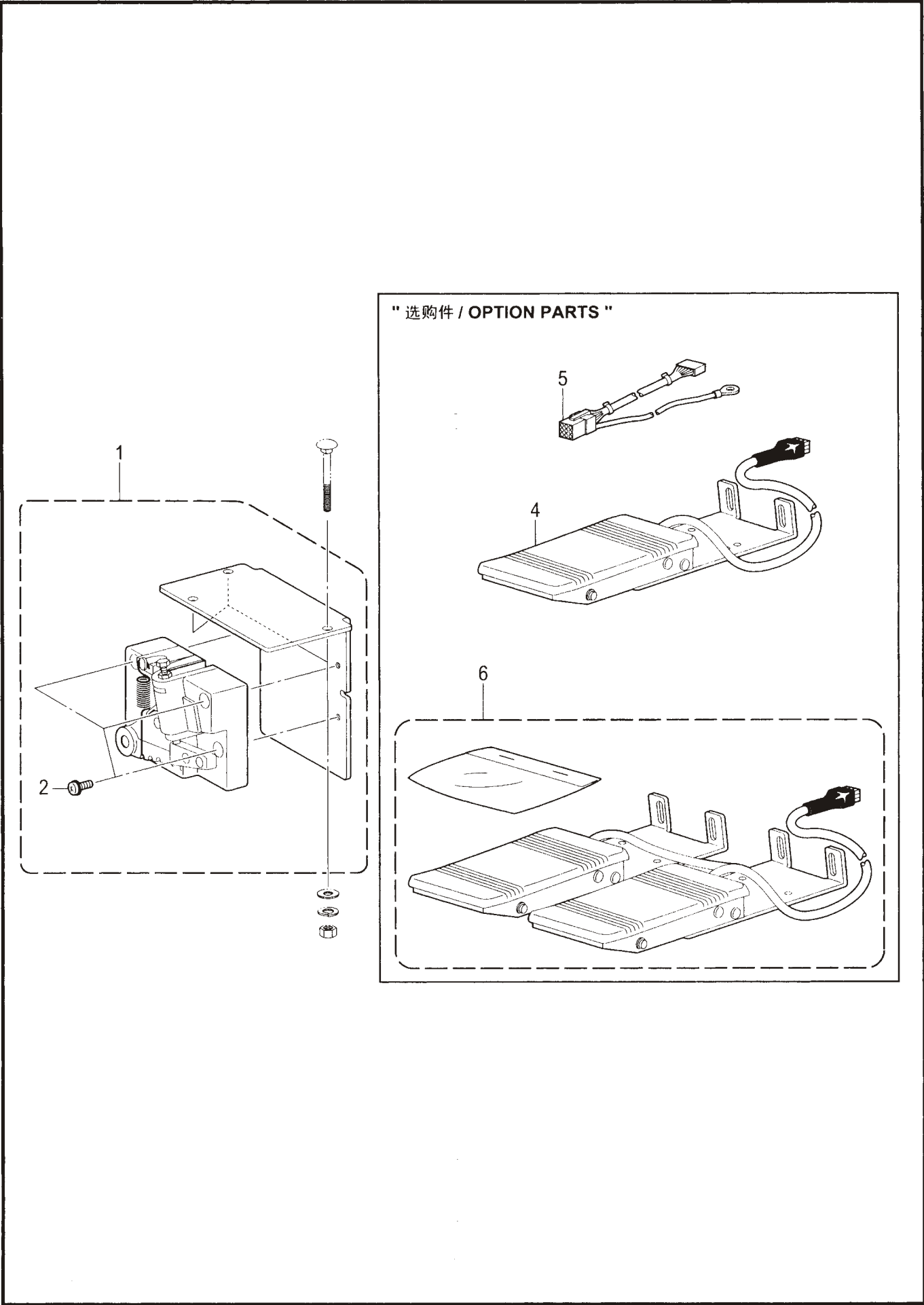
U. 踏板关系 / Foot switch pedal mechanism
