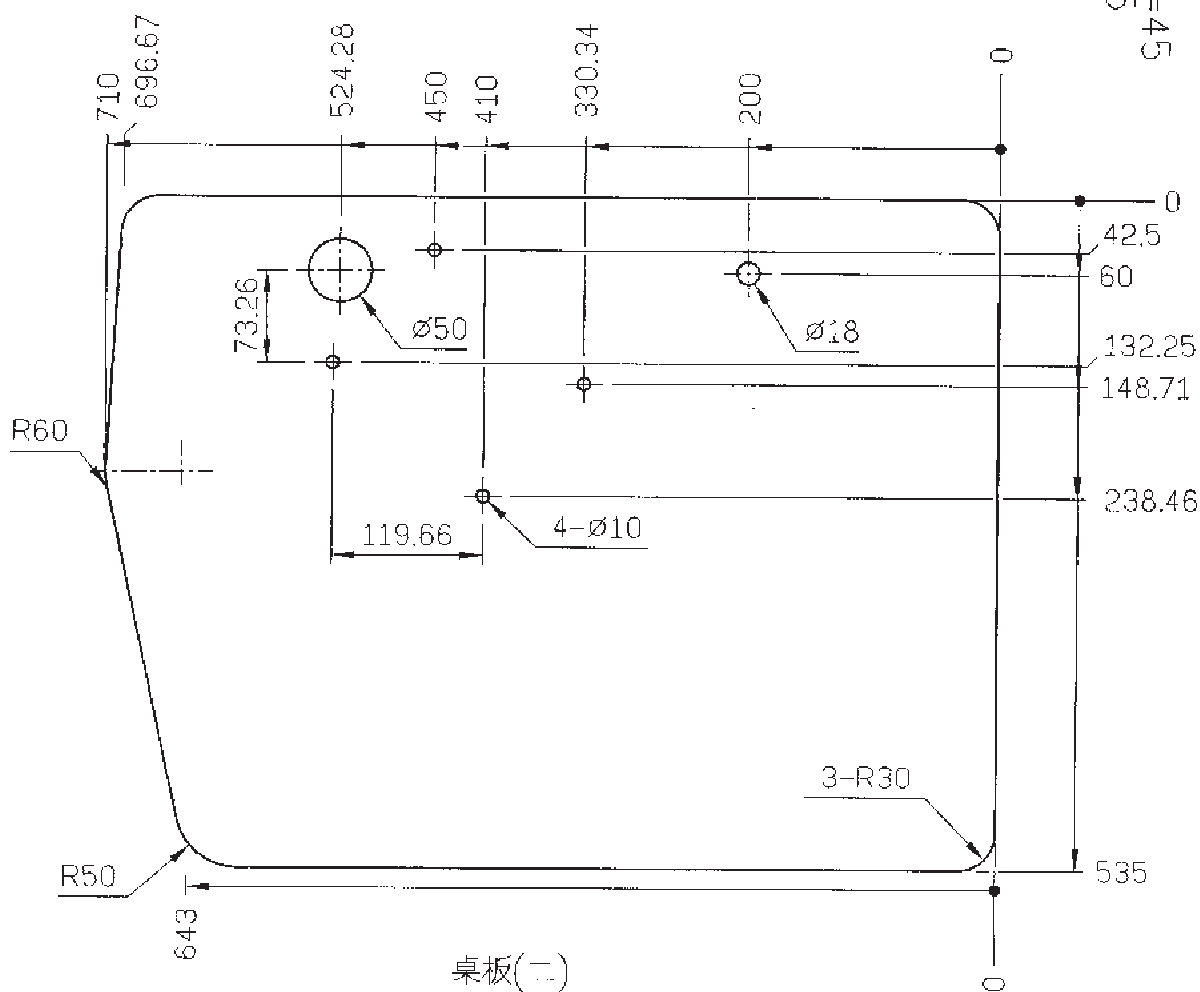
桌板(一)
